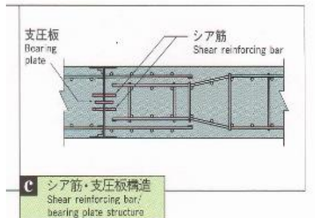
剛結継手
