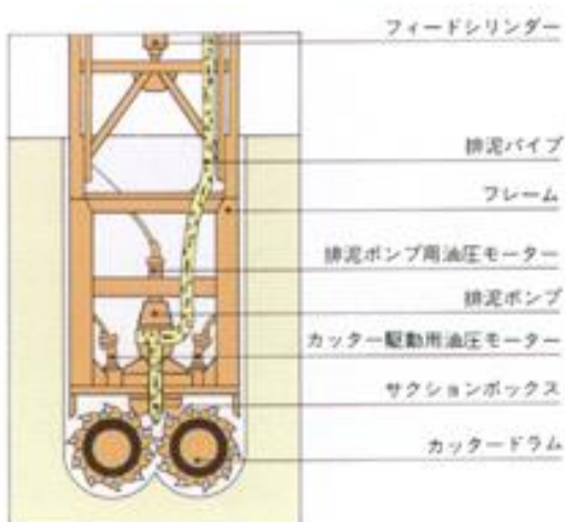
地下鉄工事(本体兼用地中連壁)
